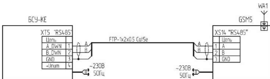
Рисунок 6 – Схема подключения для программирования адреса
