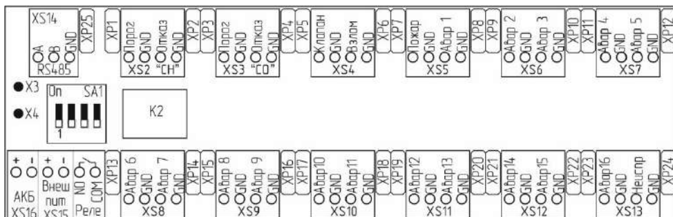
Рисунок Б.1 – Расположение элементов в клеммном отсеке
