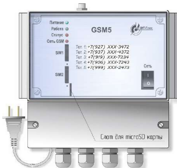
Рисунок 1 – Внешний вид извещателя
