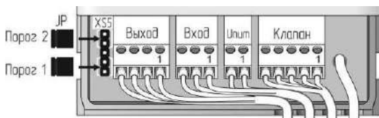
Рисунок 3 – Вид клеммного отсека C3-1-2Г
