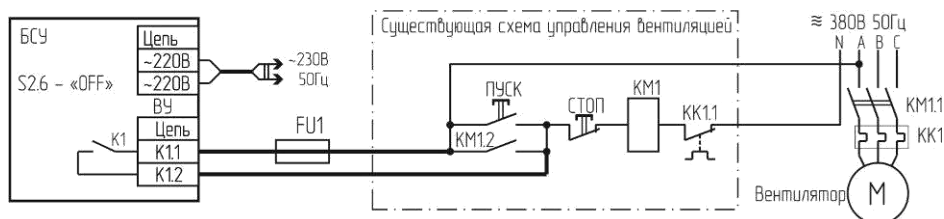
г) схема управления вентиляцией
