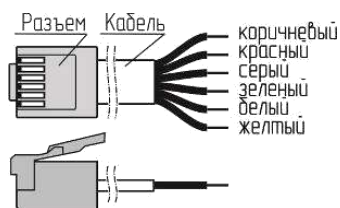
Вилка на кабель TR6P6C Нумерация проводов
