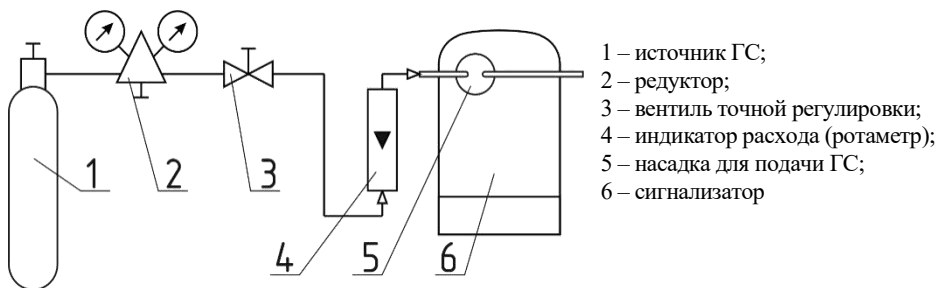
Рисунок Д.1 – Схема для настройки порогов срабатывания
