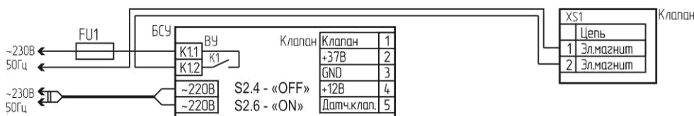
б) схема подключения клапана типа ВН
