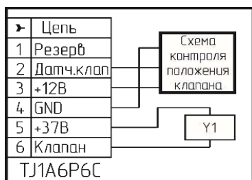
Рисунок 4 – Клапан КЗЭУГ. Схема электрическая принципиальная.
