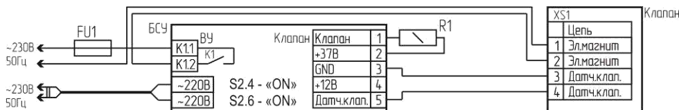
а) схема подключения клапана типа КИЭГ
