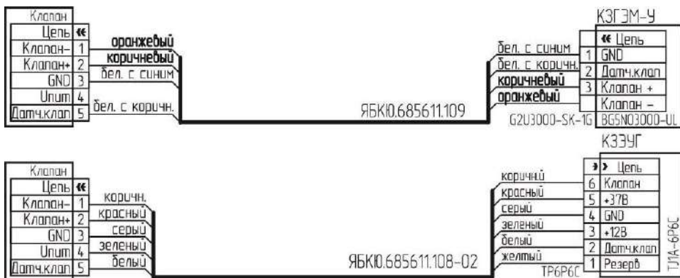
а) сигнализаторы C3-IE-485(P)/(24)
