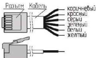
Вилка на кабель ТР6Р6С (цветовая маркировка проводов)
