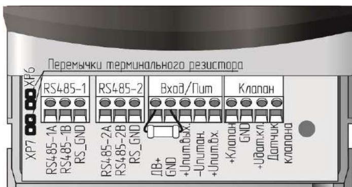
Рисунок В.3 – Расположение разъемов сигнализатора С3-1Е-485-2, С3-1Е-485Р4(Р8).
