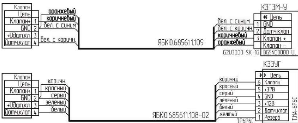
б) сигнализаторы C3-IE-485-2/(24), C3-IE-485P4(P8)/(24)
