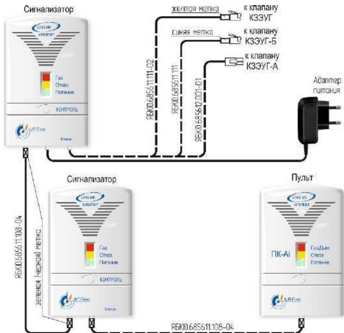
Рисунок Б.1 – Типовая схема соединений
