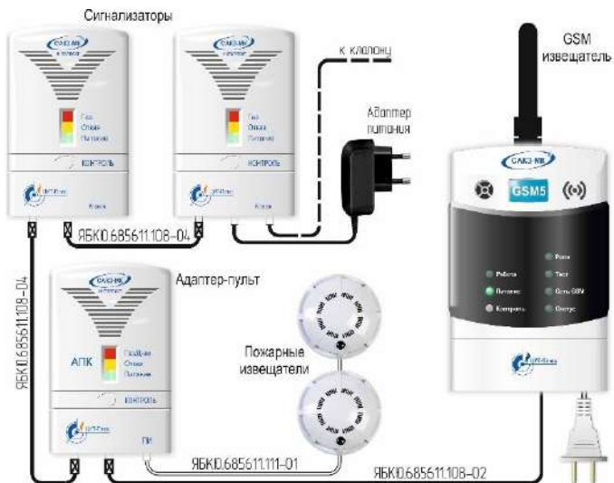
Рисунок Б.4 – Система с GSM извещателем
