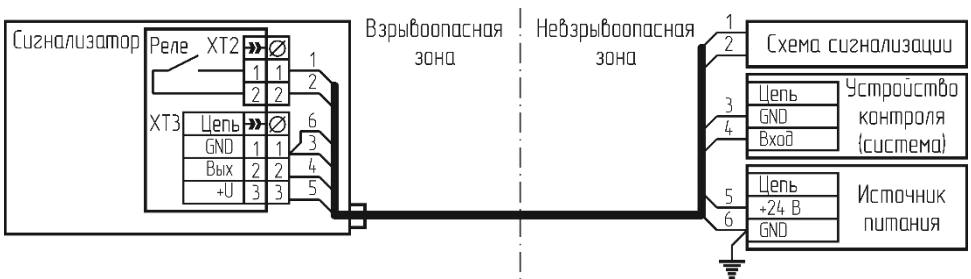
Рисунок Д.2 – Схема включения с питанием от отдельного источника
