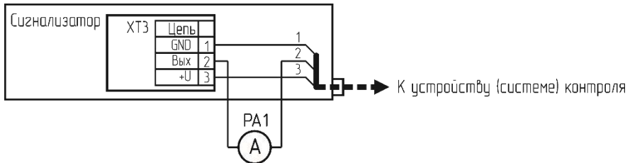
PA1 – миллиамперметр постоянного тока, шкала (0-30) мА КТ 1,5
