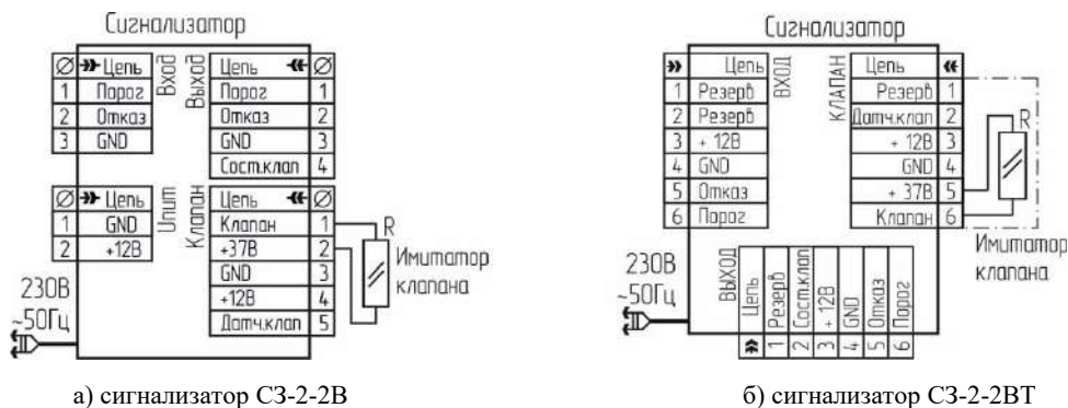
Рисунок В.1 – Типовые схемы включения сигнализаторов без клапана
