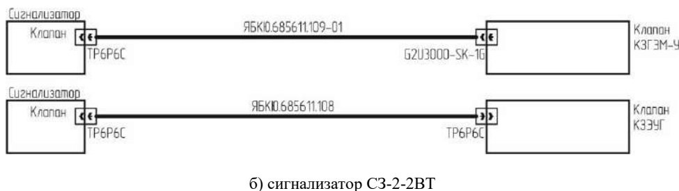
Рисунок В.3 – Схемы подключения клапанов
