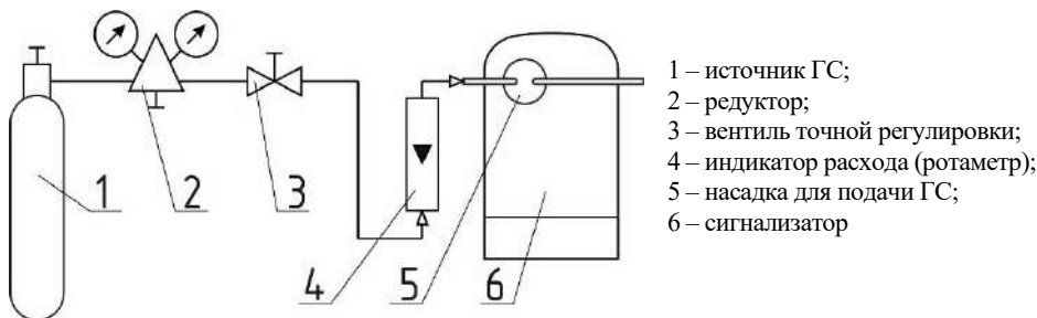
Рисунок Г.1– Схема для настройки порога срабатывания и поверки сигнализатора с применением ГС
