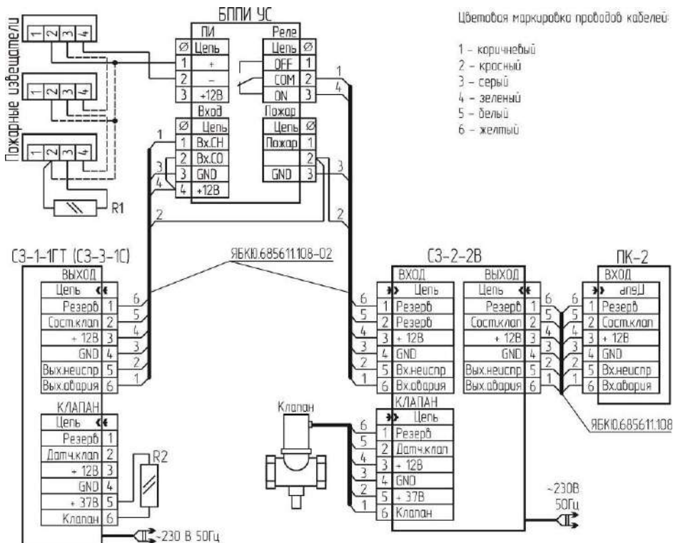
Рисунок 3 – Схема соединений с системами САЗ-МК-3, САЗ-МК-3С
