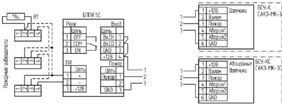
Рисунок 3 – Схема соединений с системами САЗ-МК-3, САЗ-МК-3С
