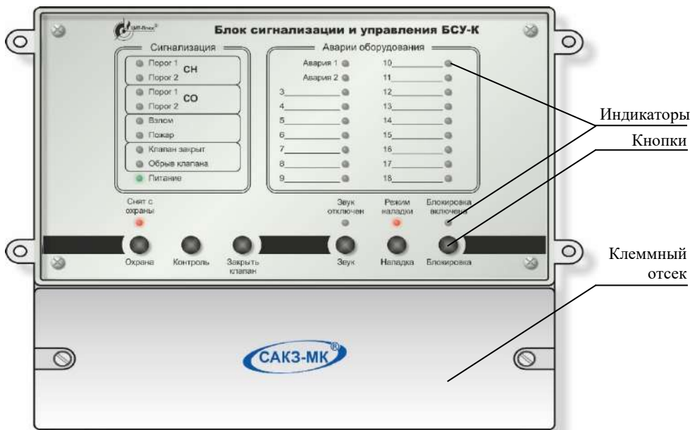
Рисунок 9 – Внешний вид БСУ-К.
