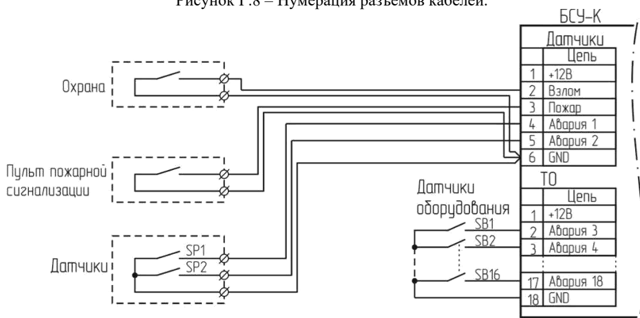
Рисунок Г.9 – Схема подключения датчиков с нормально открытыми контактами.
