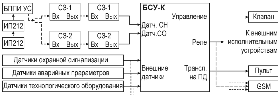
Рисунок 1 – САКЗ-МК-3. Структурная схема типовой системы
