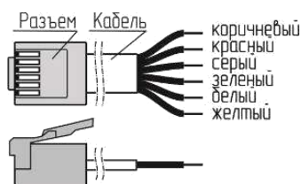
Вилка на кабель ТР6Р6С Нумерация проводов
