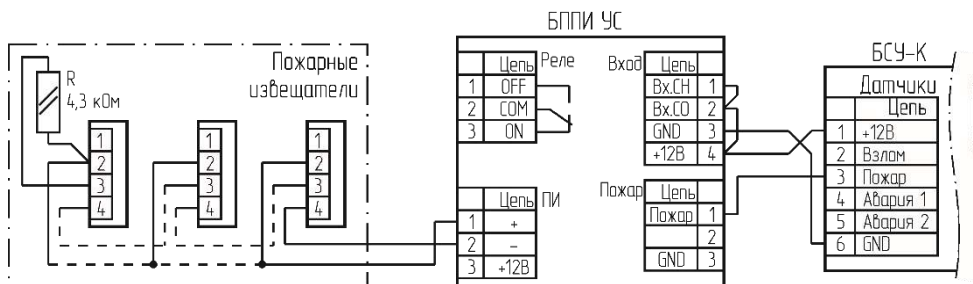
Рисунок Г.10 – Схема подключения пожарных извещателей к сигнализатору через БППИ УС.
