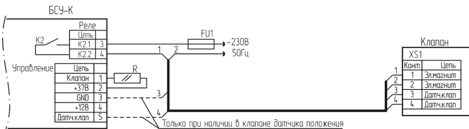
Рисунок Г.3 – Типовая схема соединений для управления вентиляцией
