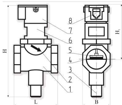
Рисунок 5 – Внешний вид клапана КЗЭУГ.
