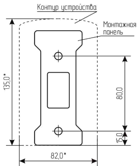
Рисунок Б.1 – Разметка отверстий для крепления сигнализаторов, пульта
