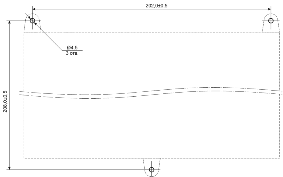
Рисунок Б.2 – Разметка отверстий для крепления БСУ-К
