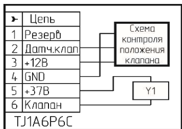
Рисунок 4 – Клапан КЗЭУГ.
