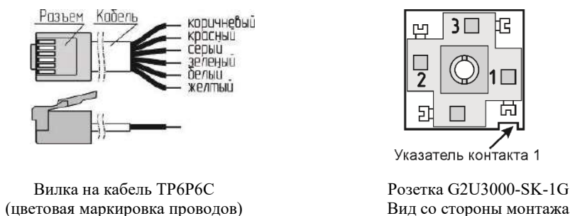
Рисунок В.5 – Нумерация контактов разъемов.
