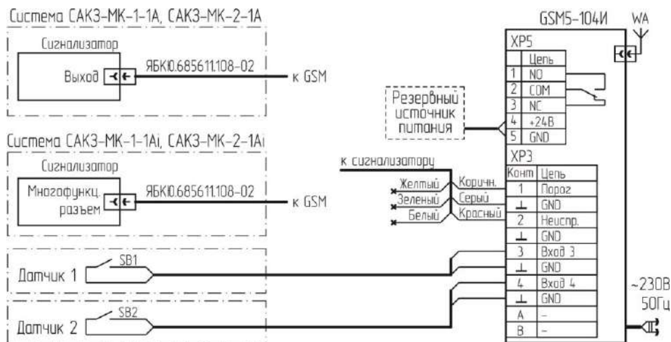
Рисунок Г.2 – Типовая схема подключения к системе САКЗ-МК-1(2)-1А(i)
