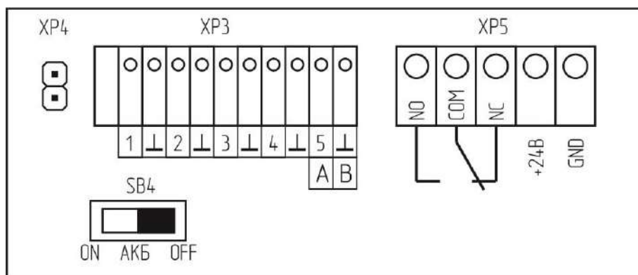
Рисунок В.1 – Расположение элементов в клеммном отсеке GSM5-104II
