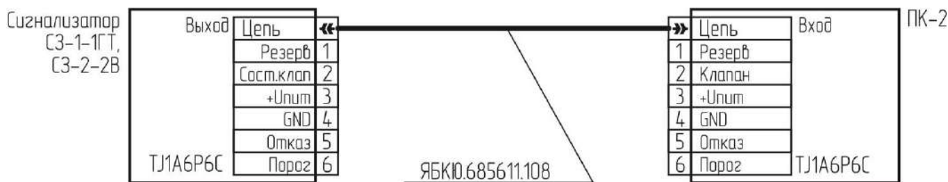
Рисунок 1 – Типовая схема подключения
